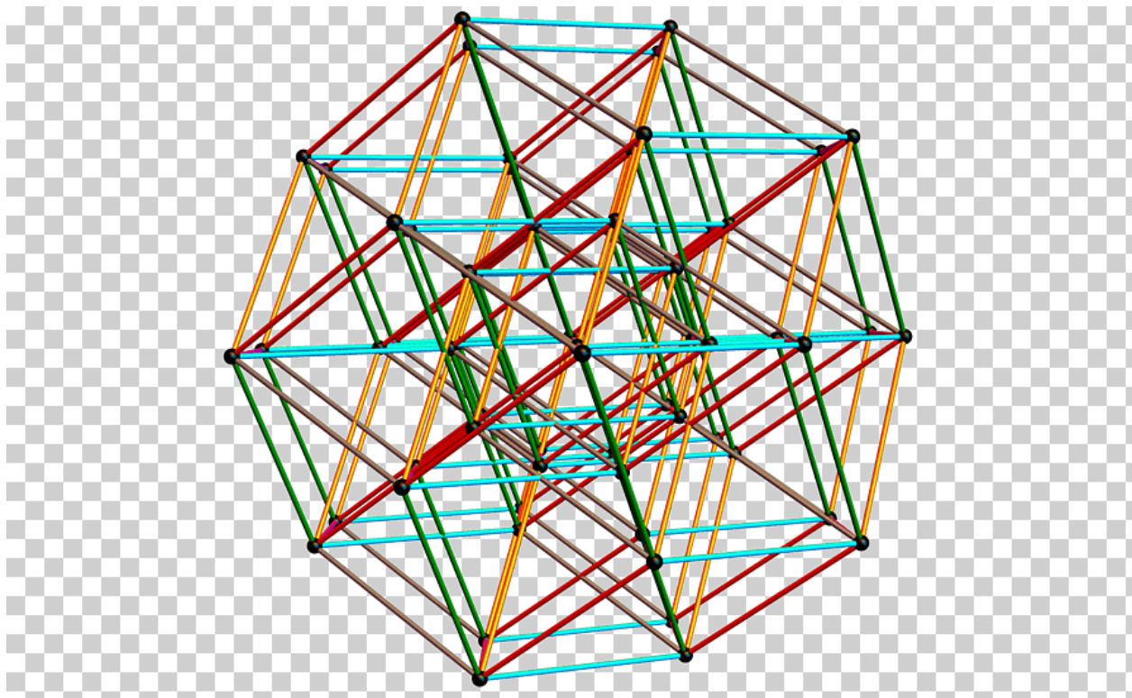
Гиперкуб
